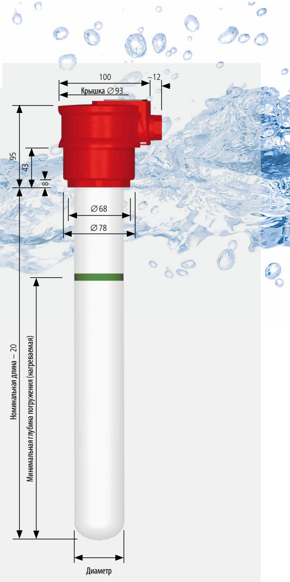
Погружные нагреватели ROTKAPPE®
